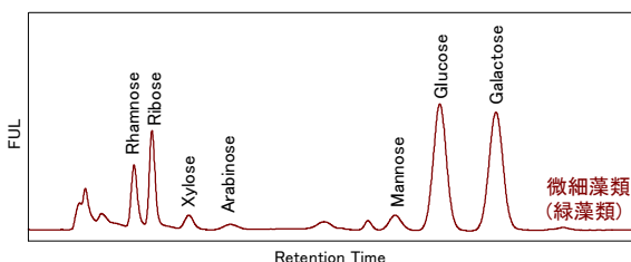
図4 藻類の中性糖HPLCクロマトグラム
