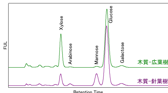
図2 木質の中性糖HPLCクロマトグラム
