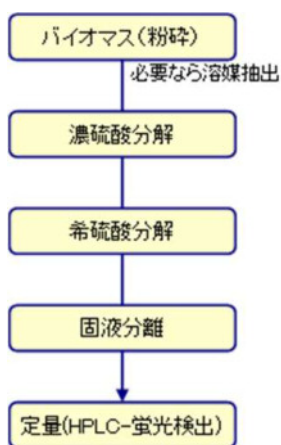
図1 分析フローチャート
