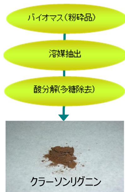
リグニン定量方法(クラークソン法)概略
